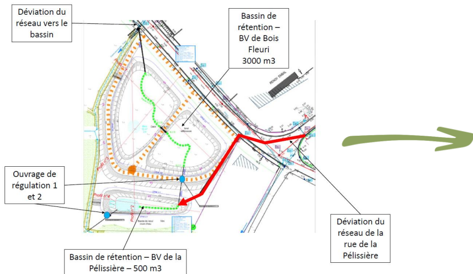
Projet de création d'un bassin pour amélioration des eaux pluviales
